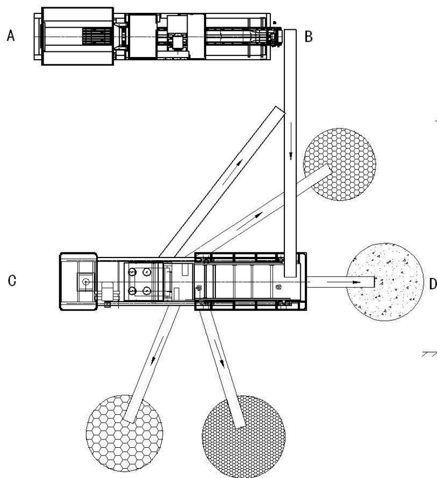
平面布置图
