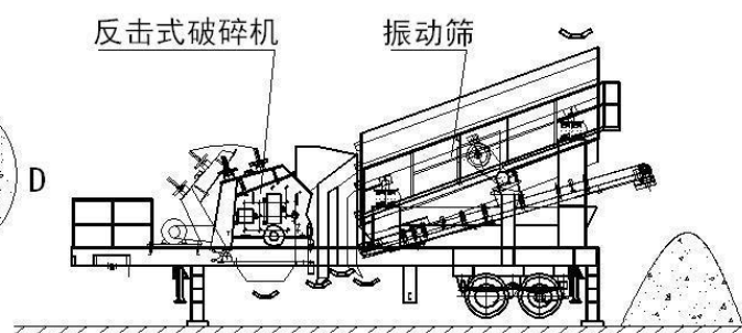
C-D段视图
