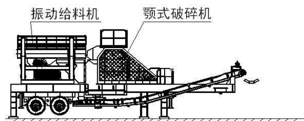
A-B段视图
